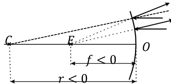
domború gömbtükör
