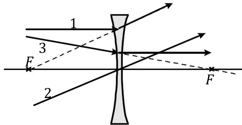
szórólencse
